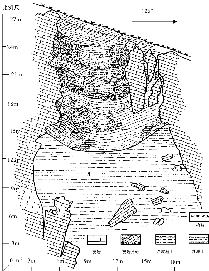
图 2 人字洞地质剖面图
